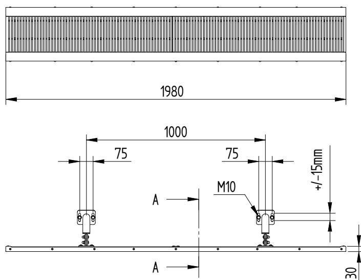
PEVNÁ OBRÁTKOVÁ STĚNA 2m
