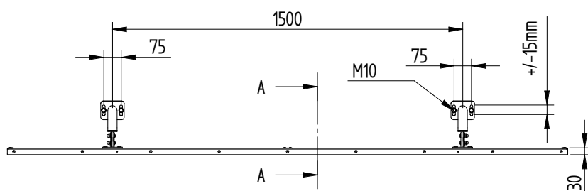
PEVNÁ OBRÁTKOVÁ STĚNA 2.5m
